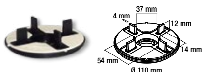
TF 2-3-4 Hlava s 2-3-4 mm spárovacími křídélky
